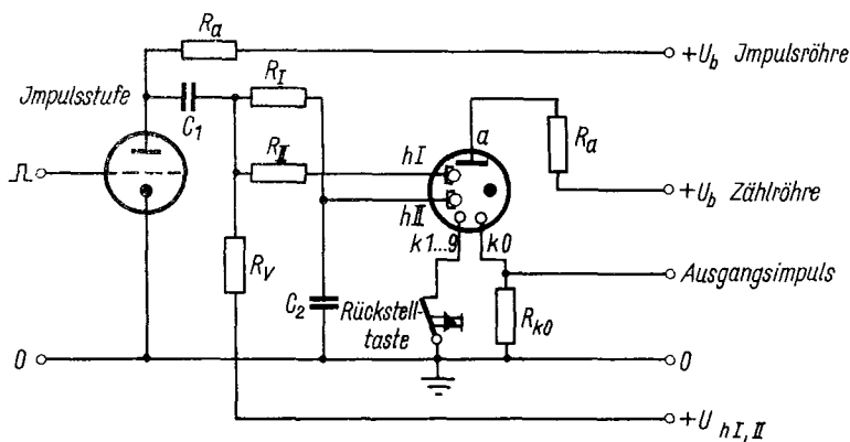
Prinzipschaltung für Steuerung durch Impulsspannungen
