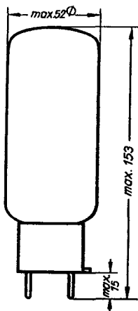
Kolbenabmessungen
