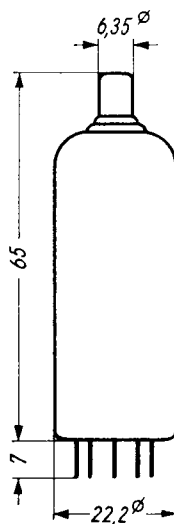
max. Abmessungen max. dimensions
