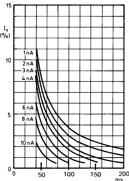
Fig. 7 XQ1410, XQ1410-L, XQ1410-G I_s/I_b = 40/600\text{nA}
