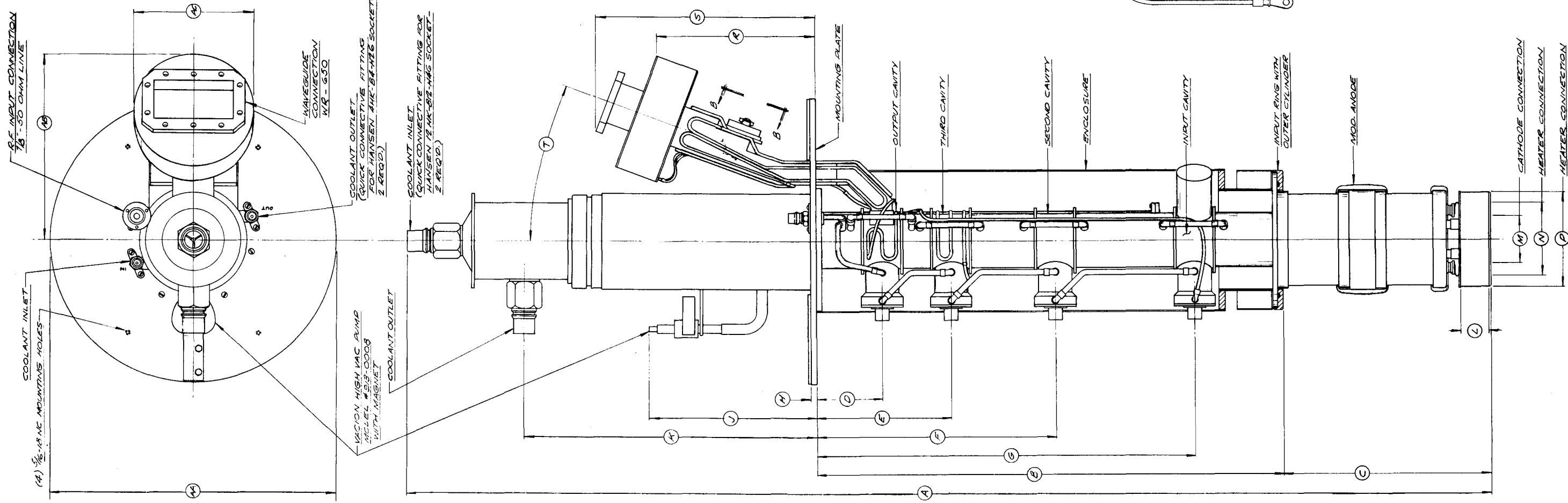
X780 KLYSTRON
