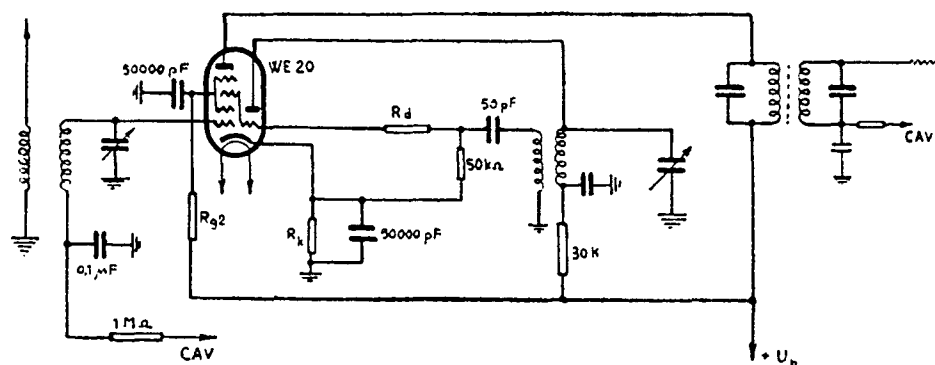
Fig. 13.44. - WE20 quale cambiafrequenza.
