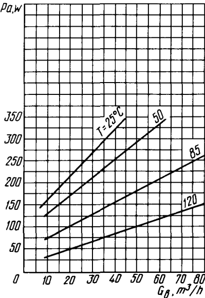
Характеристики зависимости расхода воздуха ( G_B ) от мощности, рассеиваемой анодом ( P_a ) Characteristic Curves Showing Cooling Air ( G_B ) Flow Rate versus Anode Dissipation ( P_a )
