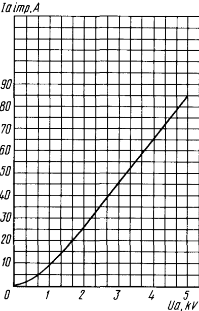
Усредненная анодная характеристика: U_i = 12,6\text{ В} Averaged Anode Characteristic Curve: U_i = 12.6\text{ V}
