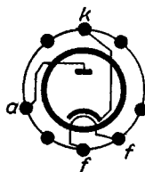
Sockelschaltschema
