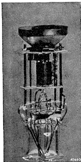
Fig. 3 Afbeelding van den elektronenstraalindicator UM 4.
