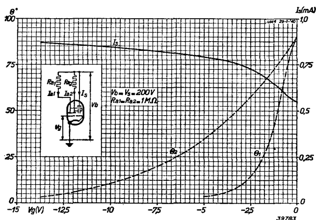
Fig. 4 Schaduwhoek \theta_1 en \theta_2 aan den rand van het scherm gemeten en schermschroom I_s als functie van de roosterspanning bij een voedingspanning van 200 V.
