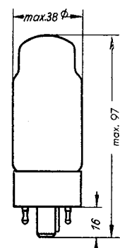
Kolbenabmessungen
