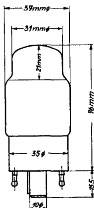
Kolbenabmessungen
