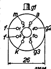
Fig. 2 Rangschikking van de elektroden en aansluitingen van de buis.
