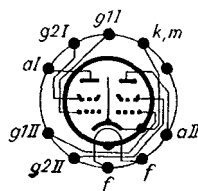
Sockelschaltschema Sockelnase nach unten
