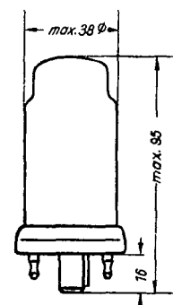
Kolbenabmessungen
