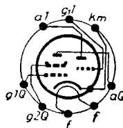
Sockelschaltschema
