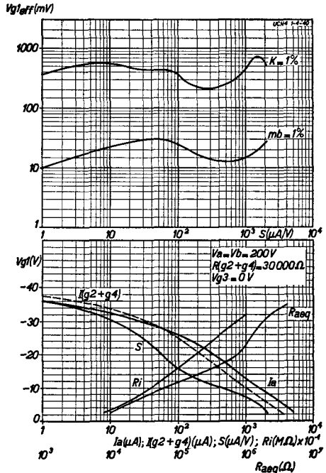
Fig. 13 7-449 Bovenste krommen: De hoogst toelaatbare effectieve waarde van de H.F. wisselspanning voor 1% kruismodulatie ( K = 1\% ) en de hoogst toelaatbare wisselspanning voor 1% modulatiebrom ( mb = 1\% ), beide van het storende signaal op het rooster, als functie van de steilheid, bij voeding van het schermrooster via een weerstand van 30\,000\,\Omega , vanuit de voedingspanning van 200\,V . Onderste krommen: Steilheid S , anodestroom I_a , schermroosterstroom I(g_2 + g_4) , inwendige weerstand Ri en equivalente ruischweerstand Raeg , als functie van de neg. roosterspanning.
