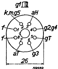
Fig. 2 Rangschikking van de electrodensystemen en aansluitingen van de huls.
