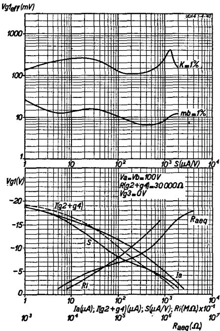
Fig. 12 39539 Bovenste krommen: De hoogst toelaatbare effectieve waarde van de H.F. wisselspanning voor 1% kruismodulatie ( K = 1\% ) en de hoogst toelaatbare wisselspanning voor 1% modulatiebrom ( mb = 1\% ), beide van het storende signaal op het rooster, als functie van de steilheid, bij voeding van het schermrooster via een weerstand van 30\,000\,\Omega , vanuit de voedingspanning van 100\,V . Onderste krommen: Steilheid S , anodestroom I_a , schermroosterstroom I(g_2 + g_4) , inwendige weerstand Ri en equivalente ruischweerstand Raeg , als functie van de neg. roosterspanning.
