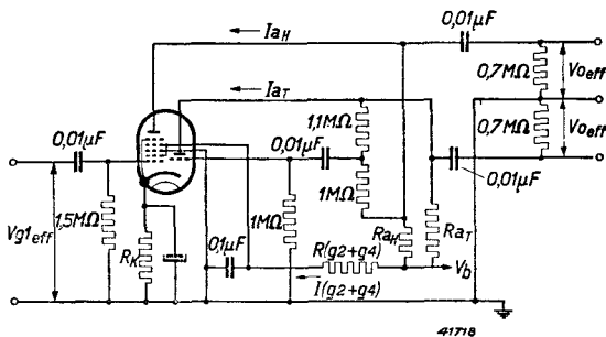
Fig. 16 Principieele schakeling van de UCH 4 als fase-omkeerbuis met tegenkoppeling.
