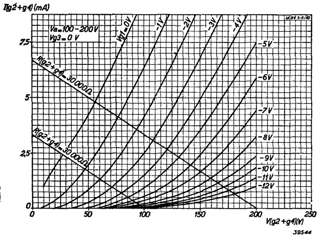
Fig. 14 Schermroosterstroom als functie van de schermroosterspanning bij V_a = 100-200\,V en V_{g3} = 0\,V met V_{g1} als parameter.
