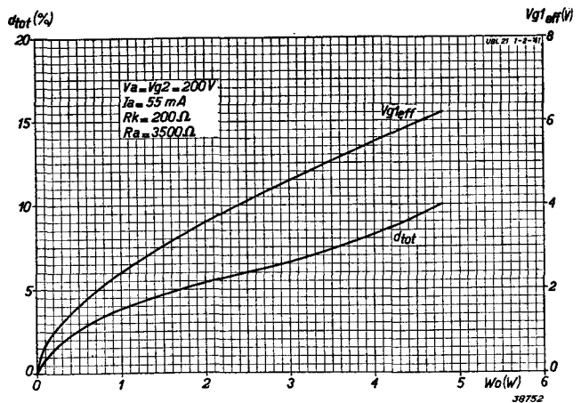
Fig. 9 Totale vervorming en vereichte roosterwisselspanning als functie van het geleverde vermogen, bij V_a = V_{g2} = 200 \text{ V} en R_a = 3500 \Omega .
