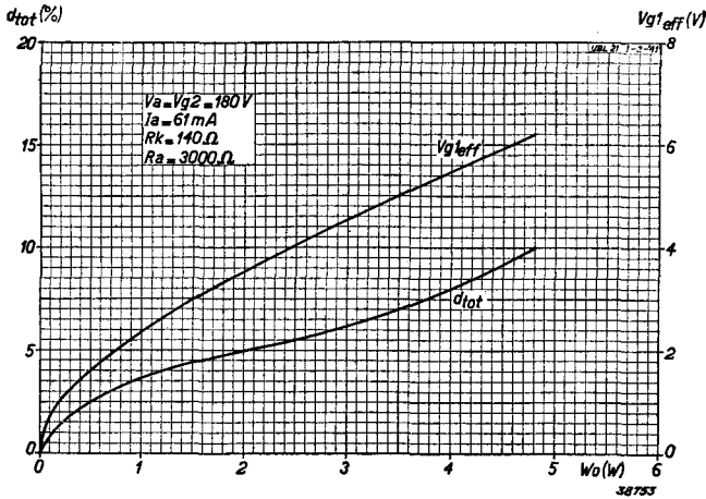
Fig. 8 Totale vervorming en vereichte roosterwisselspanning als functie van het geleverde vermogen, bij V_a = V_{g2} = 180 \text{ V} en R_a = 3000 \Omega .
