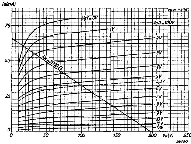
Fig. 4 Anodestroom als functie van de anodespanning bij V_{g2} = 100 \text{ V} met V_{g1} als parameter; de belastinglijn voor R_a = 3000 \Omega is tevens in deze grafiek getekend.
