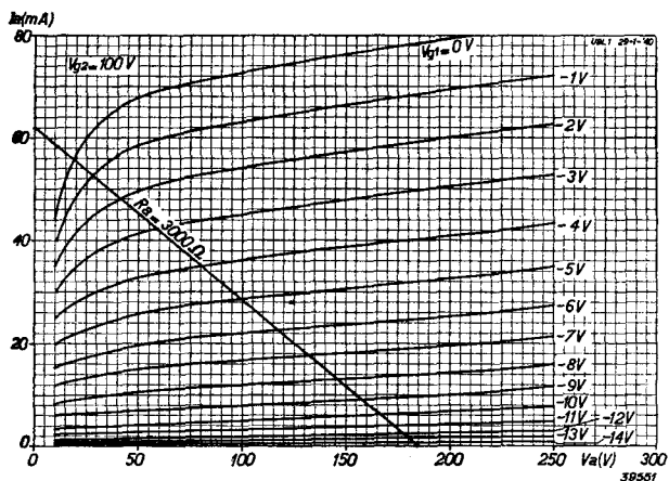
Fig. 4 Anodestroom als functie van de anodespanning bij V_{g2} = 100V en met V_{g1} als parameter.
