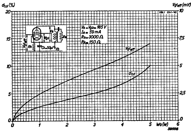
Fig. 8. Totale vervorming en vereichte roosterwisselspanning als functie van het geleverde vermogen bij V_a = V_{g2} = 185 \text{ V} .
