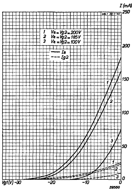
Fig. 3 Anode- en schermroosterstroom als functie van de negatieve roosterspanning bij V_a = V_{g_2} = 200 V, 185 V en 100 V.
