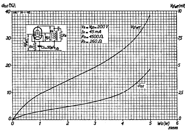
Fig. 9 Totale vervorming en vereichte roosterwisselspanning als functie van het geleverde vermogen bij V_a = V_{g2} = 200 \text{ V} voor de 9 W instelling.
