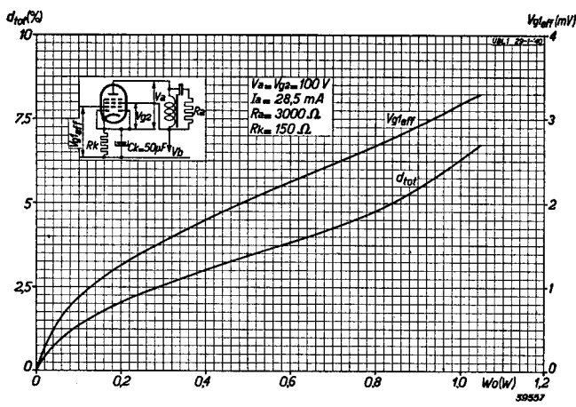
Fig. 7 Totale vervorming en vereichte roosterwisselspanning als functie van het geleverde vermogen bij V_a = V_{g2} = 100 \text{ V} .
