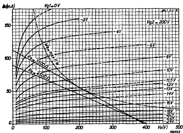
Fig. 6 Anodestroom als functie van de anodespanning bij V_{g2} = 200V en met V_{g1} als parameter. De belastinglijnen voor de 9 W instelling ( R_a = 4500\Omega ) en de 11 W instelling ( R_a = 3500\Omega ) zijn tevens in deze grafiek getekend.
