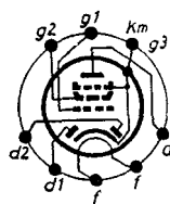
Sockelschaltschema
