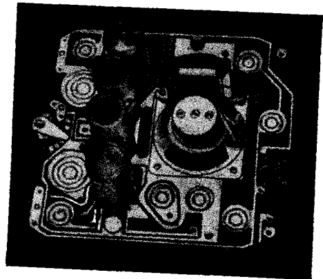
Tweekringler met 2 stuks UA-55, daar tussen in twee electrolieten.
