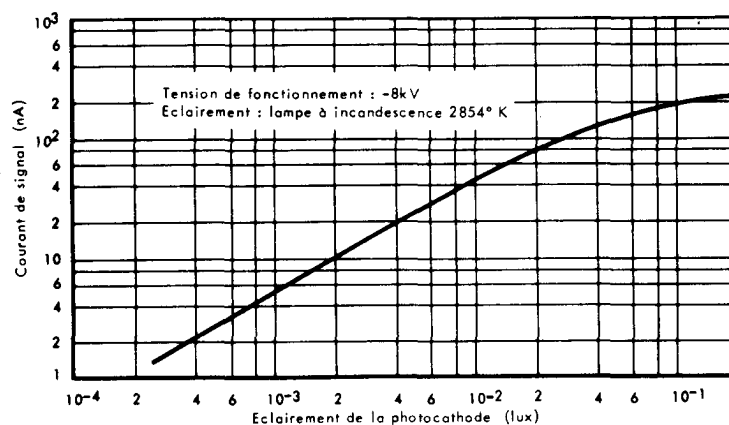
Fig 2 - Caractéristique signal - éclaïrement .
