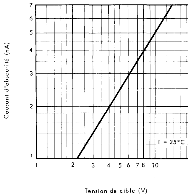
Figure 3 - Caractéristique de courant d'obscurité.
