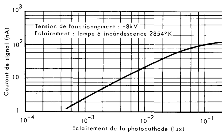
Fig 2 - Caractéristique signal-éclairage
