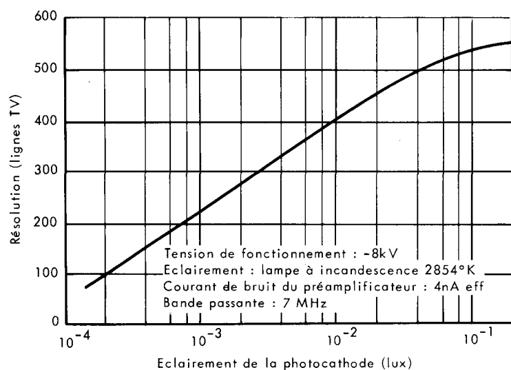
Fig 4 - Résolution statique en fonction de l'éclairement de la photocathode
