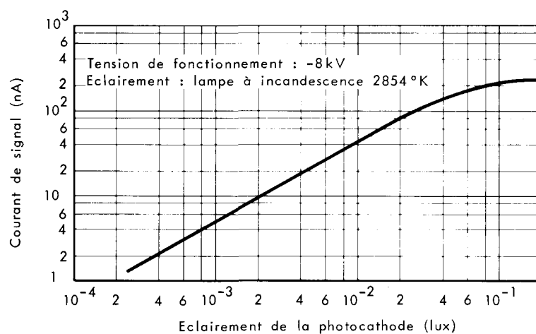
Fig. 2 - Caractéristiques signal - éclairage.
