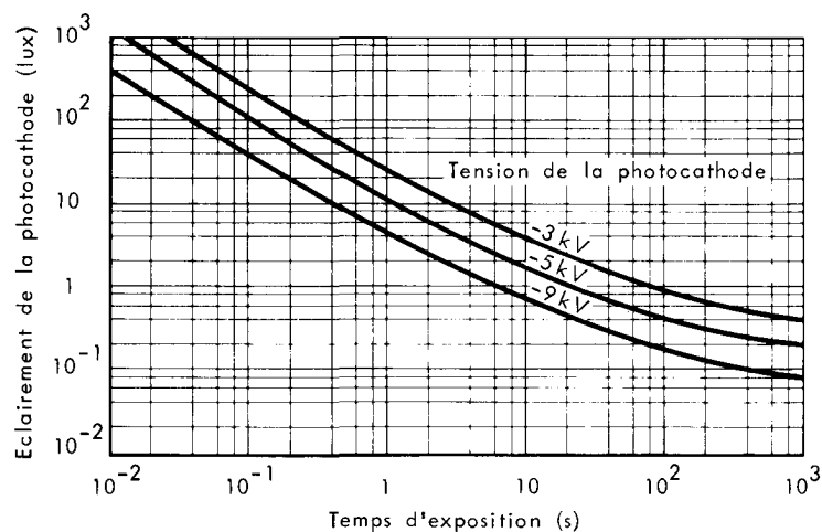
Fig. 1 - Eclairements limites.
