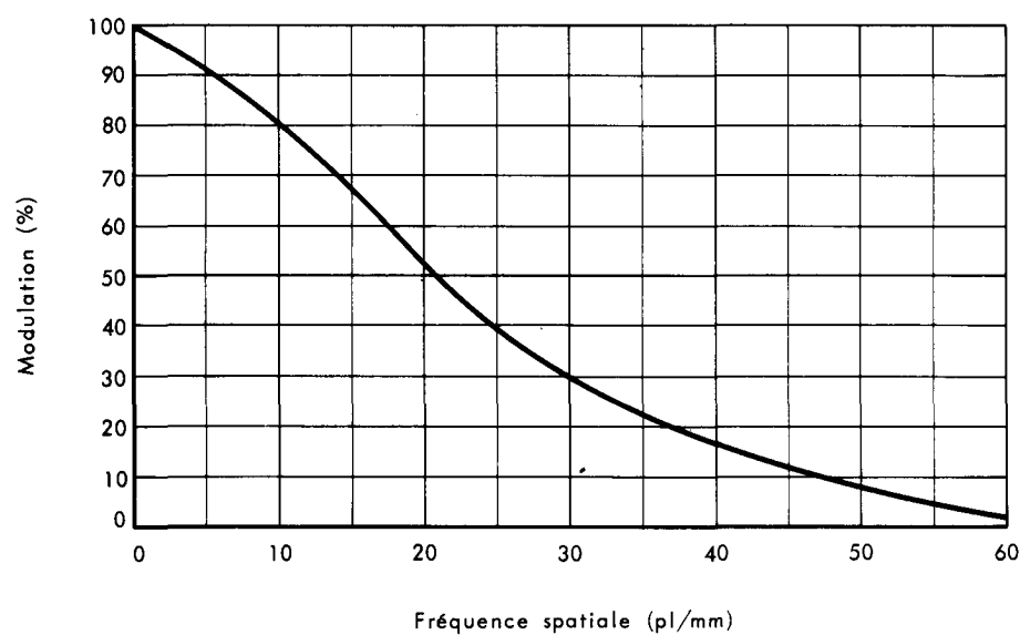
Fig. 4 - FTM mesurée au niveau de la photocathode (valeurs typiques)
