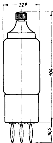
max. Abmessungen
