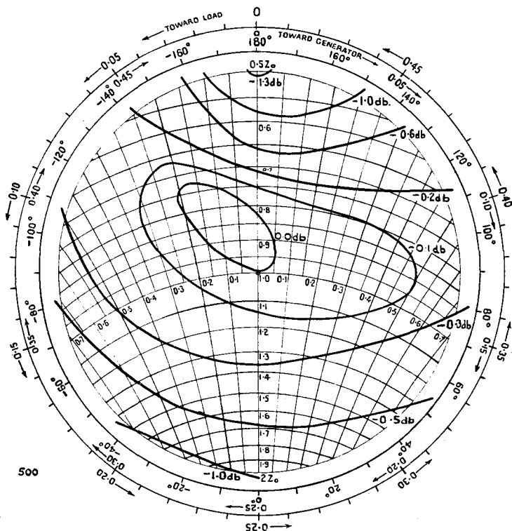
RIEKE DIAGRAM.
