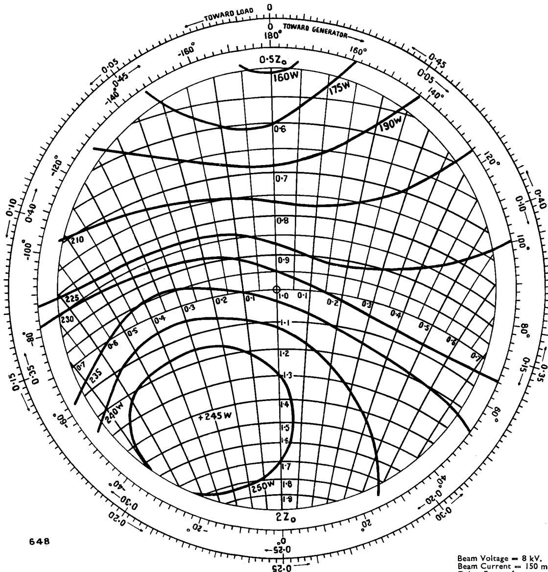
RIEKE DIAGRAM
