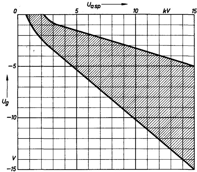
Zündkennlinienstreubereich
