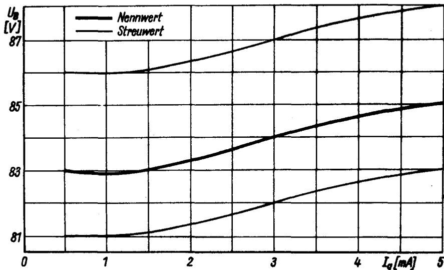
Brennspannungskennlinie
