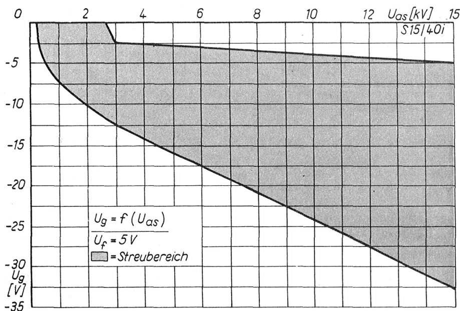
Zündkennlinien-Streubereich
