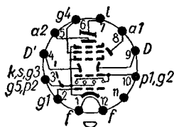
Sockelschaltenschema
