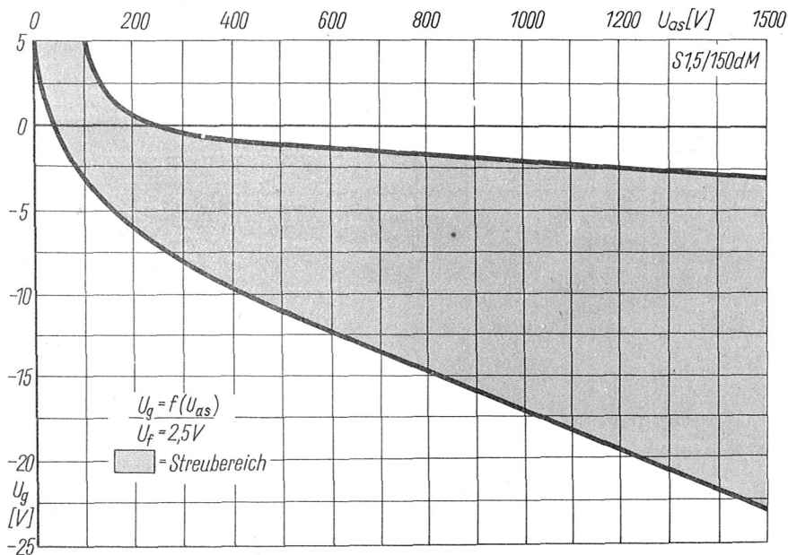
Zündkennlinien-Streubereich
