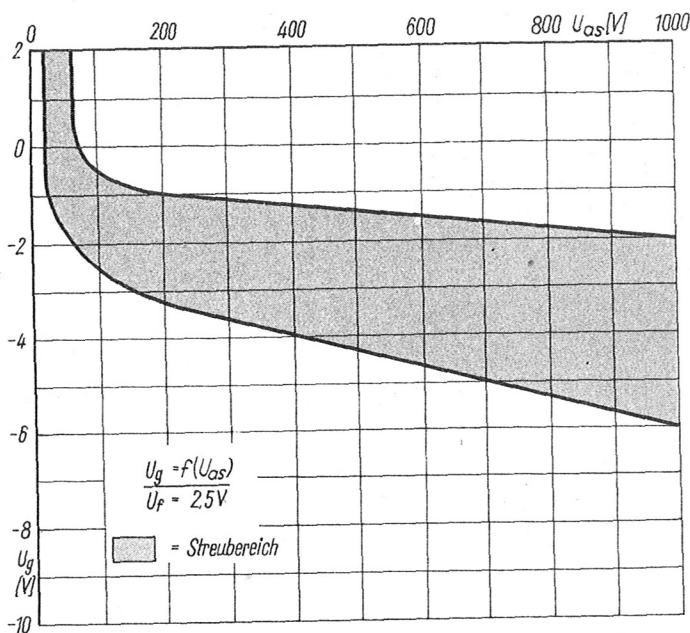
Zündkennlinien-Streubereich
