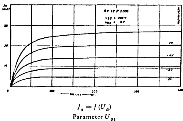
Kennlinienfelder für die Verwendung in NF-End- und Senderstufen.
