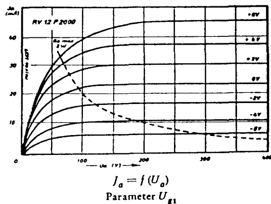
Kennlinienfelder für die Verwendung in NF-End- und Senderstufen.
