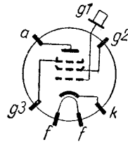
Sockelschaltenschema
