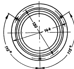
Einwandkühltopf Lg.-Nr. 30356
