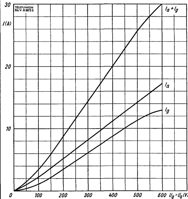
Emissionskennlinien
