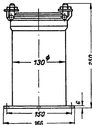
Doppelwandkühltopf Lg.-Nr. 30355
