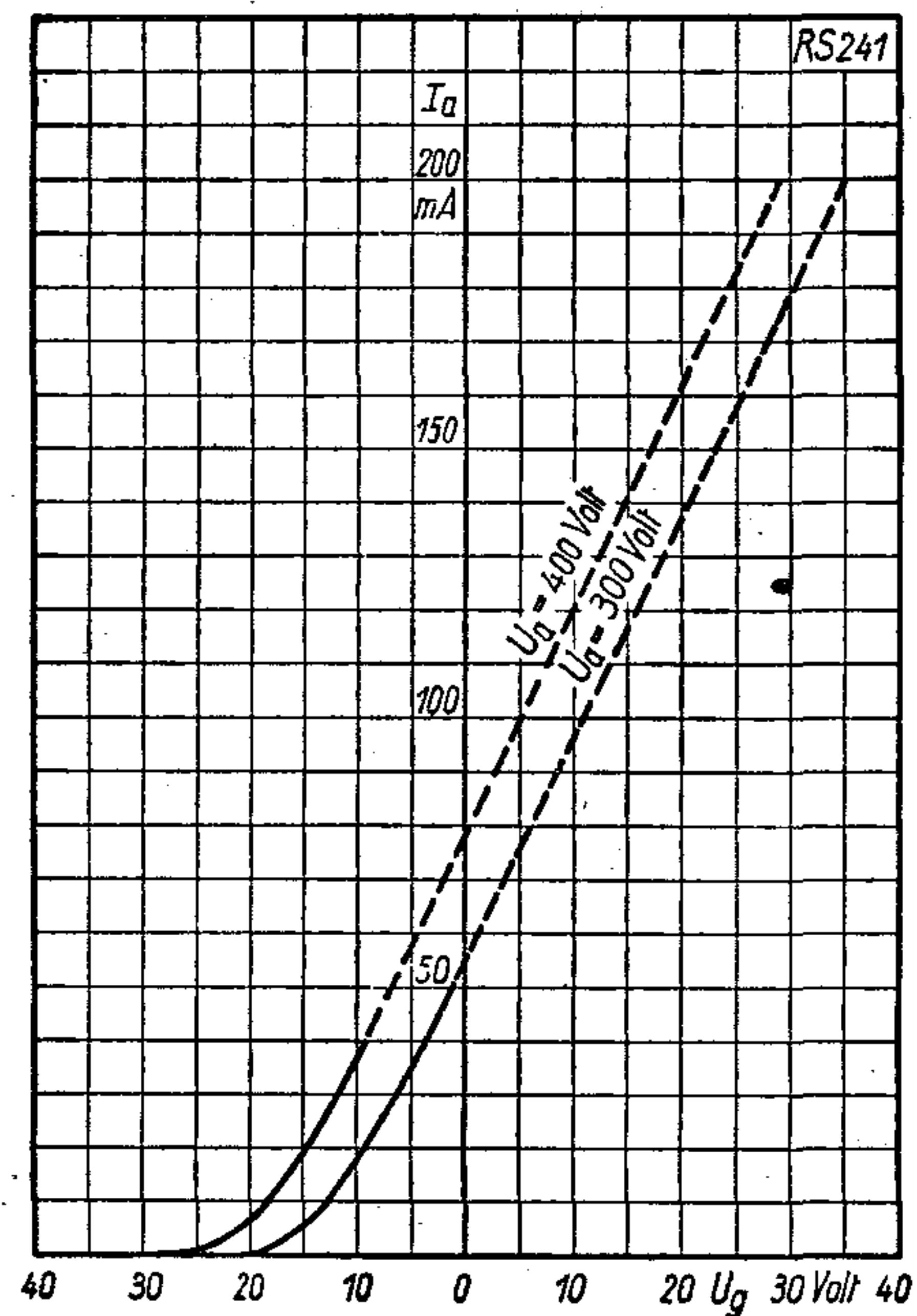
Statische Kennlinie
