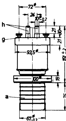
Ausführung für Wasserkühlung RS 2011 W
