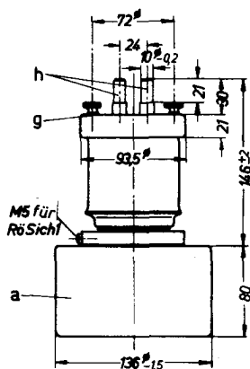
Ausführung für Luftkühlung RS 2011 L
