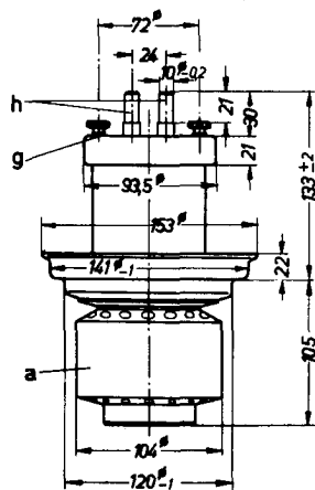
Ausführung für Verdampfungskühlung RS 2011 V
