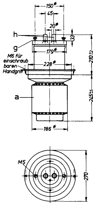
Ausführung für Verdampfungskühlung RS 2001 K YD 1032
