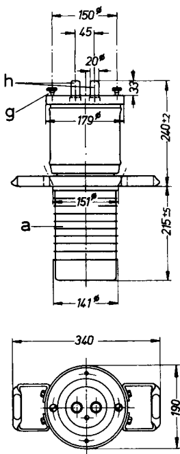
Ausführung für Wasserkühlung RS 2001 W YD 1030
