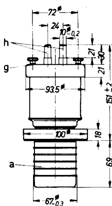
Ausführung für Wasserkühlung RS 1061 W
