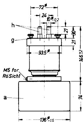
Ausführung für Luftkühlung RS 1061 L
