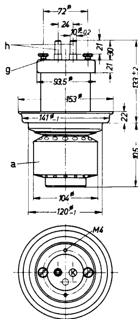
Ausführung für Verdampfungskühlung RS 1061 V
