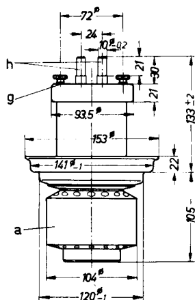
Ausführung für Verdampfungskühlung RS 1061 V
