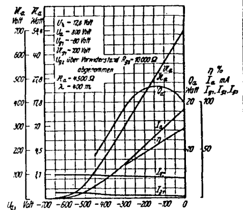
Bremsgittermodulation bei U_a = 800 V
