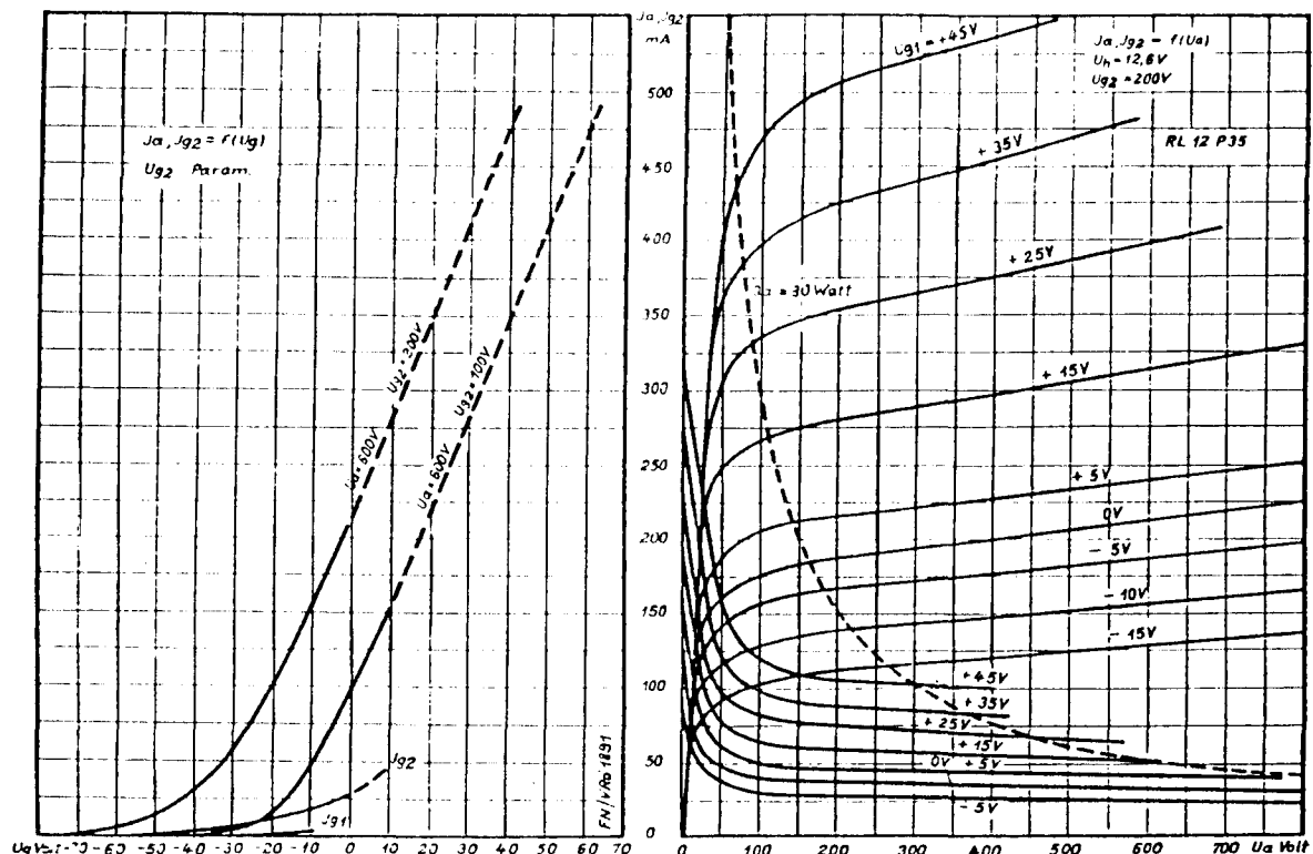
Statisches Kennlinienfeld
