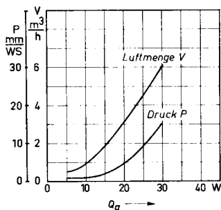
Kühlluftdiagramm
