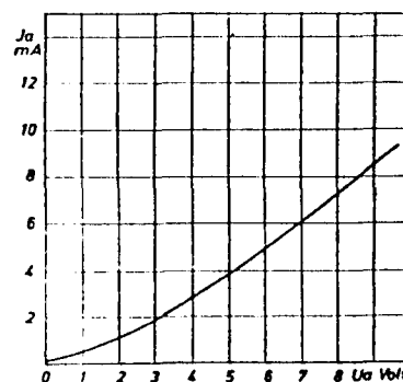
I_a - U_a -Kennlinie im Raumladungsgebiet
