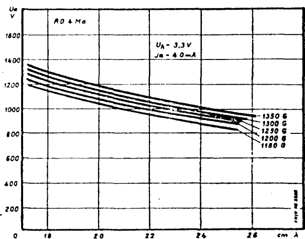
Schwingkennlinien
