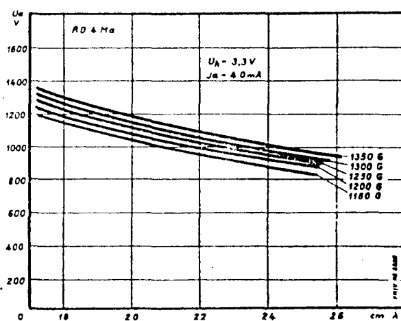
Schwingkennlinien
