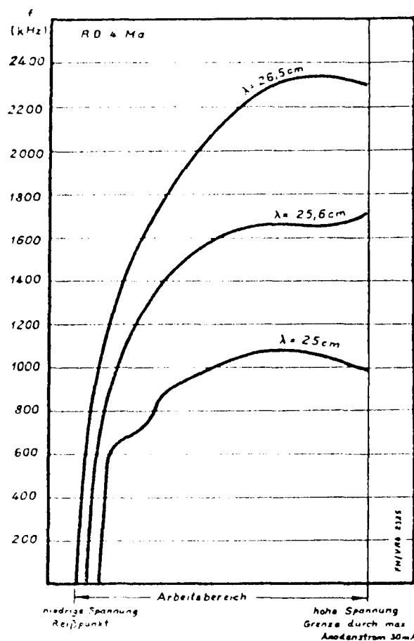
Änderung der Frequenz in Abhängigkeit von der Anodenspannung
