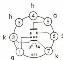
B7G Base
