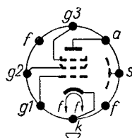
Sockelschaltsschema
