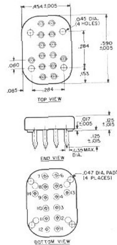
RTS-44 SOCKET
